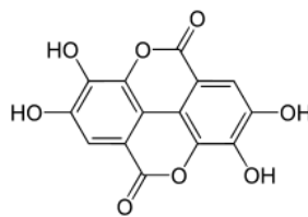
ელაგის მჟავა
